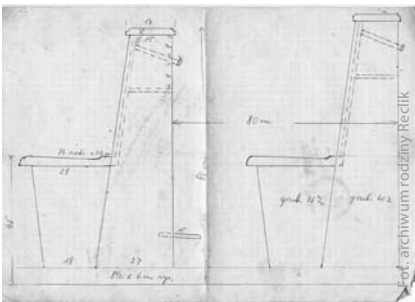
Schemat budowy ławek kościelnych
